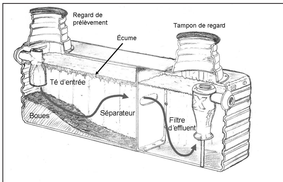
Figure 2 Vue en coupe d'une fosse septique courante avec regards de prélèvement et filtre d'effluent
