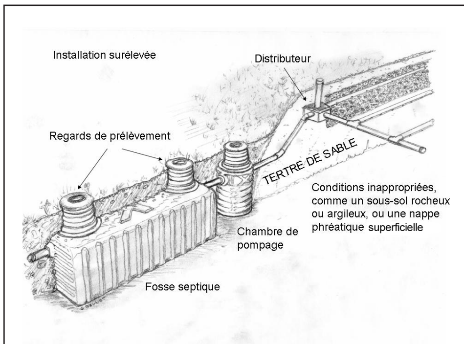
Figure 4 Installation surélevée
