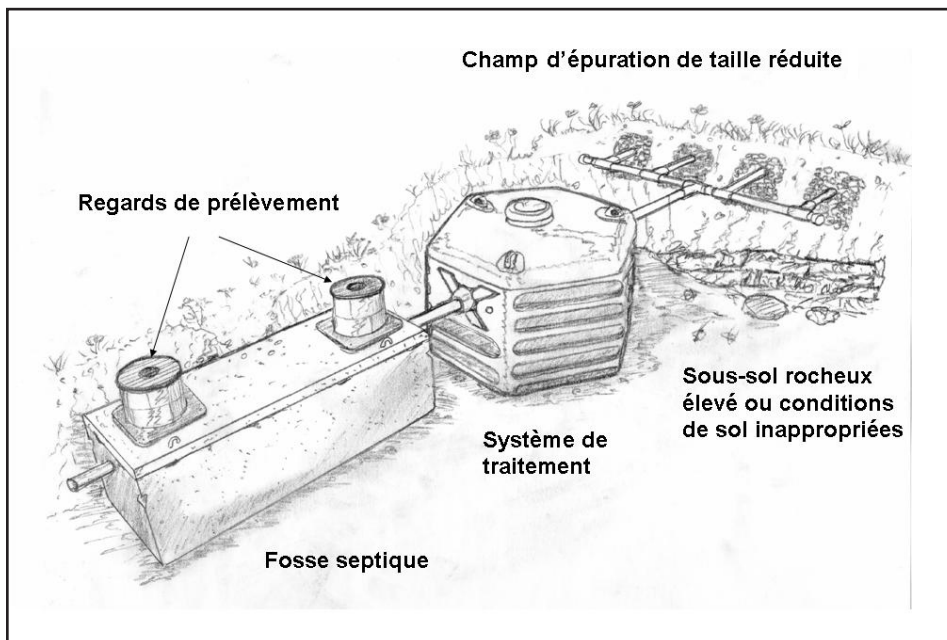
Figure 5 Autre technique de traitement
