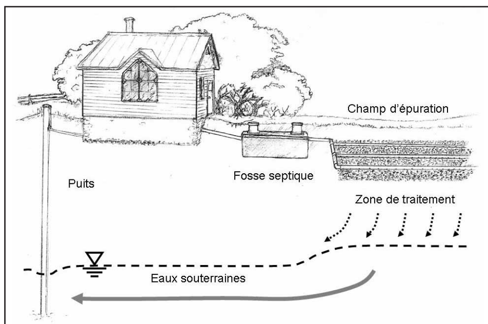
Figure 1 Recyclage des eaux usées par une installation autonome
